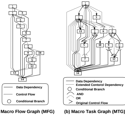
図 1 マクロフローグラフ (MFG)、マクロタスクグラフ (MTG) の例
