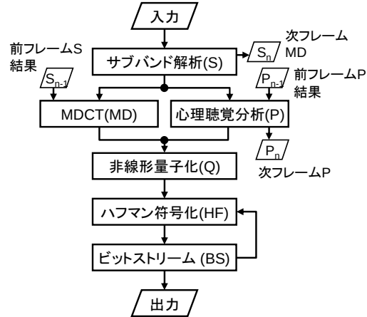
図 5 MP3 の処理フロー
