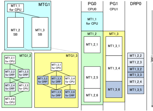
図 3 スケジューリングの例
