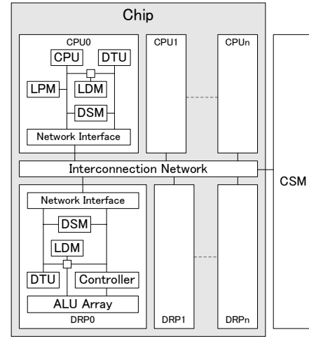
図 2 OSCAR 型メモリアーキテクチャを持つヘテロニアスチップマルチプロセッサの例
