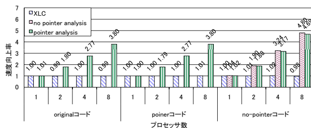
図 4 art の速度向上率
