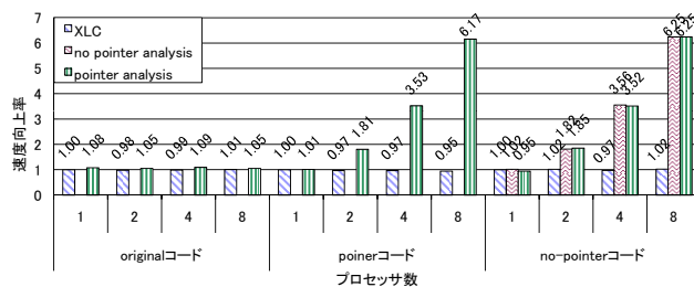
図 5 lbm の速度向上率
