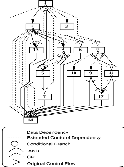
図 2: マクロフローグラフの例
